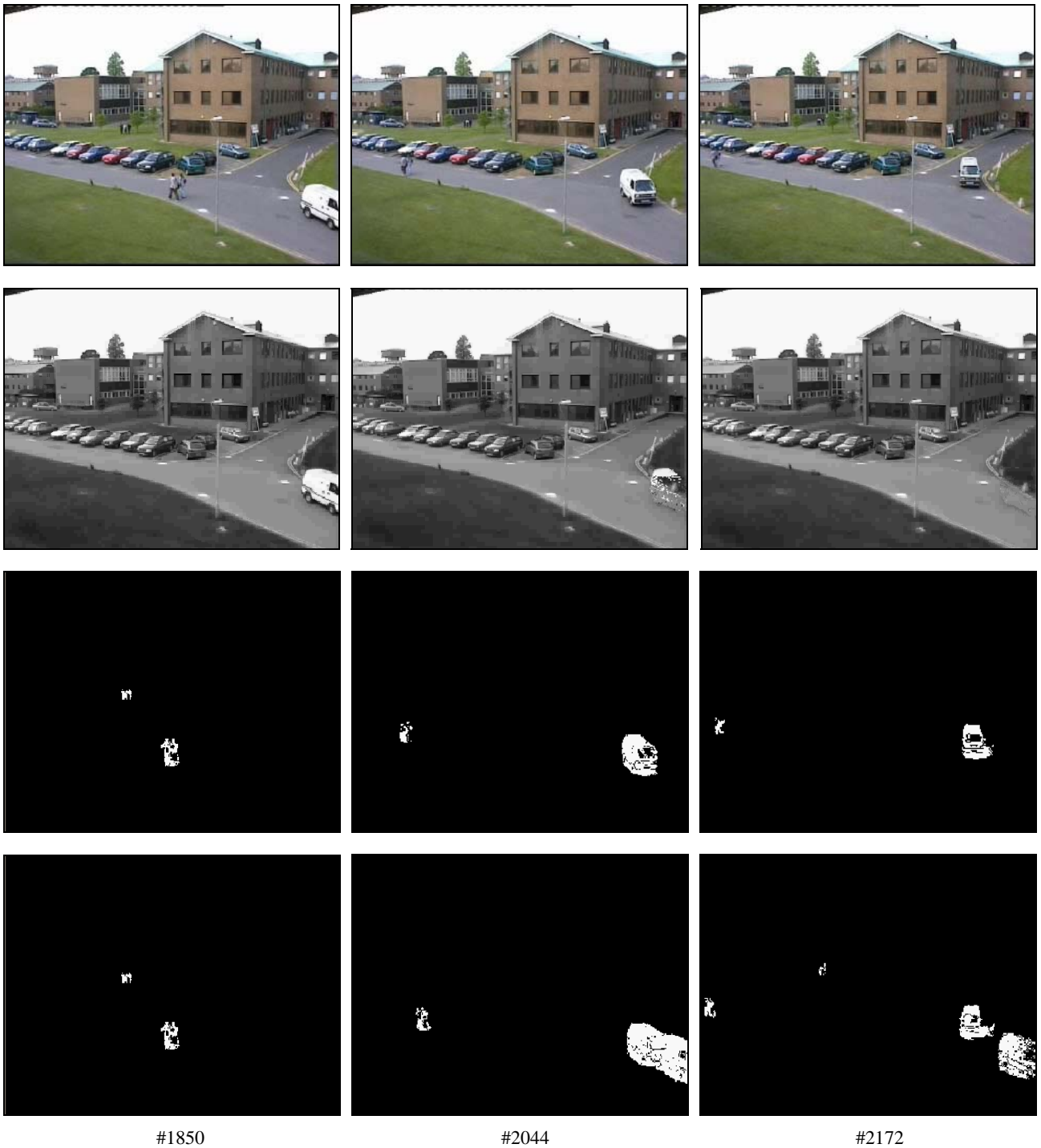
图 2 PETS 2002 数据库运动前景检测结果比较。第一行：输入视频序列；第二行：MLBM 的动态背景；第三行：MLBM 的前景检测结果；第四行：C.Stauffer 的混合高斯背景模型 [10] 的前景检测结果。
