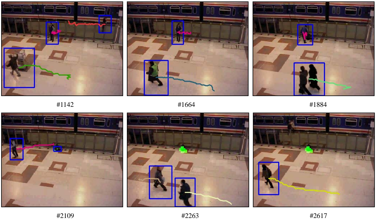
图 3 PETS 2006 数据库遗留物品检测与运动目标跟踪测试结果。检测到的遗留物品在图中用绿色显示 (#2263, #2617)，蓝色矩形框表示检测到的运动目标，彩色曲线表示目标轨迹。
