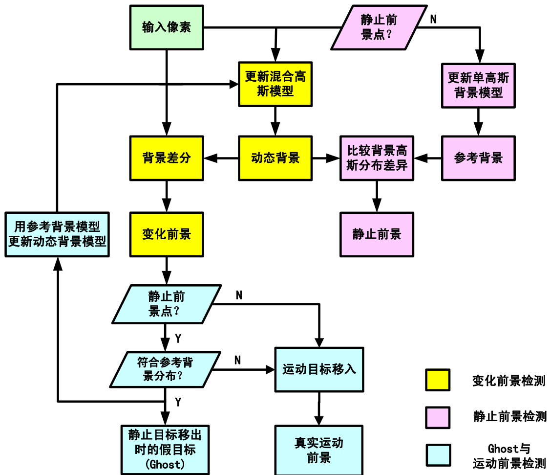
图 1 基于多层背景模型的前景检测算法框图
